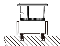
Рис. 5 Схема врезной установки кнопки
